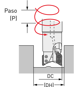
2.2 Agujeros pasantes
